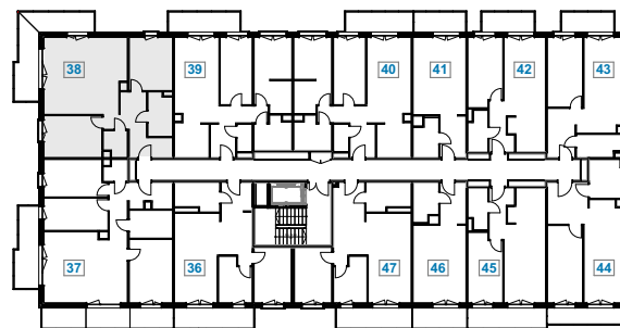
RZUT KONDYGNACJI
